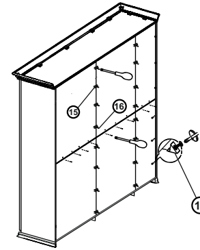
Установка петли
